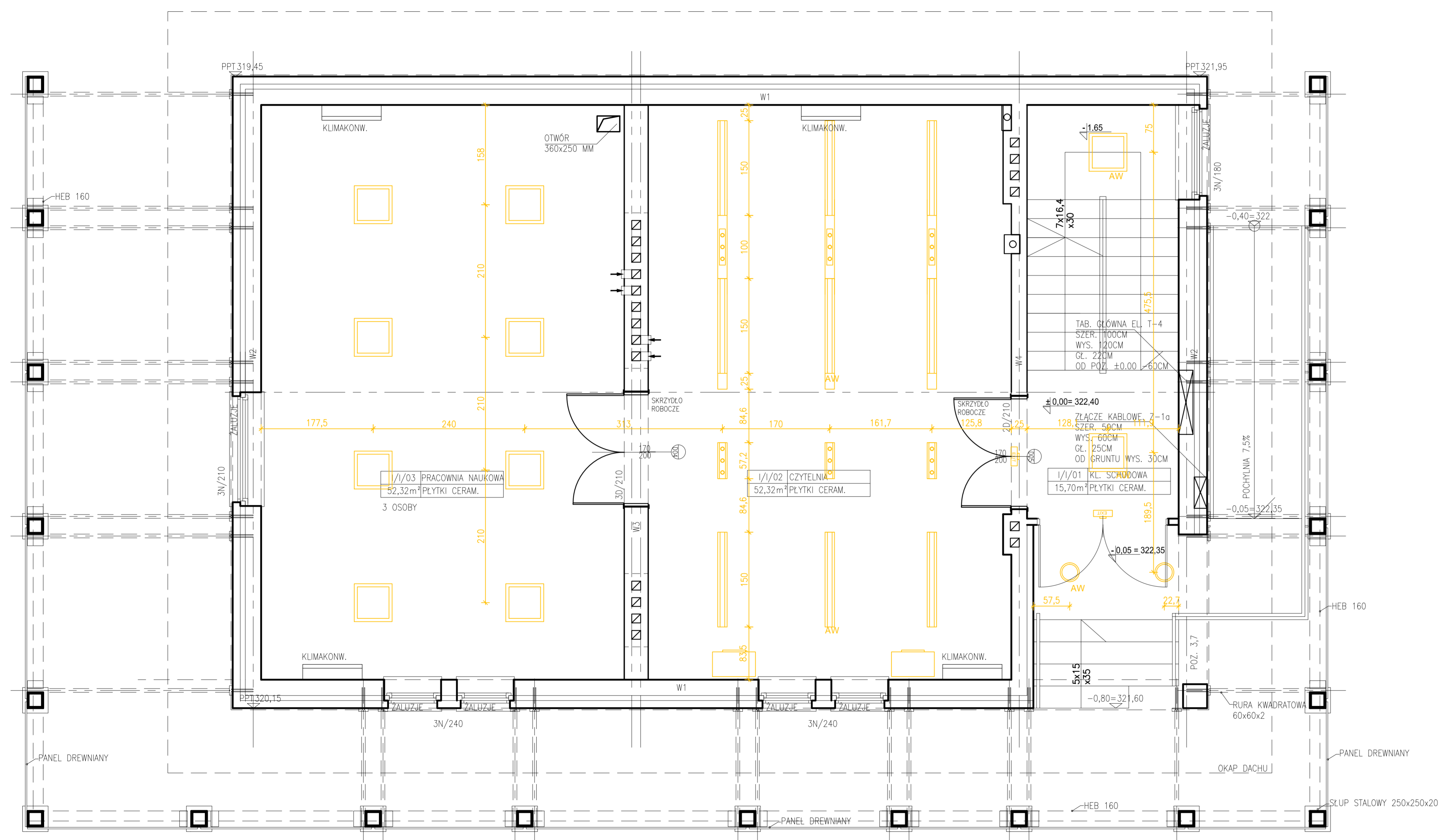
RZUT OŚWIETLENIA
